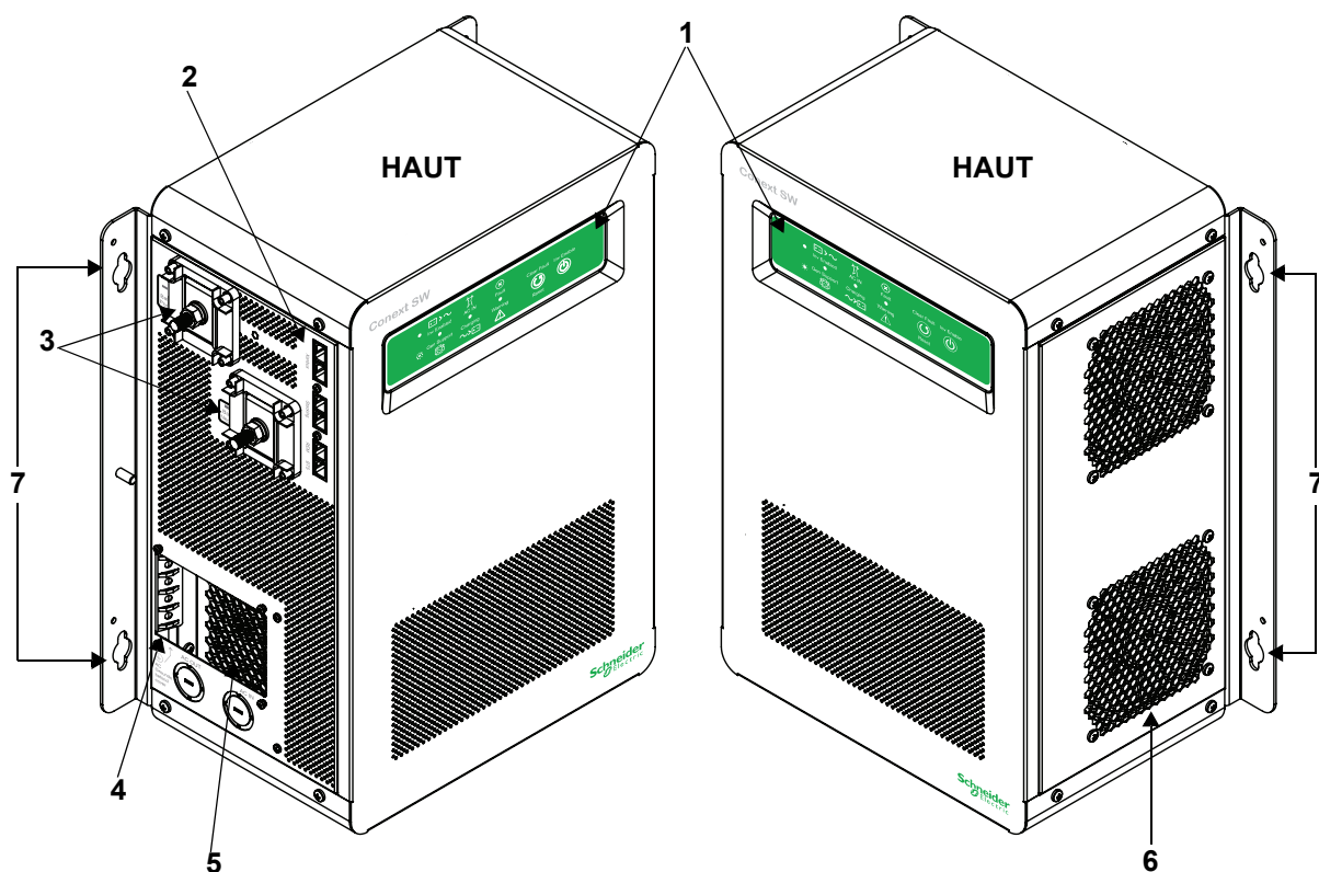
Figure 2-2 Faces avant et latérale du Conext SW
