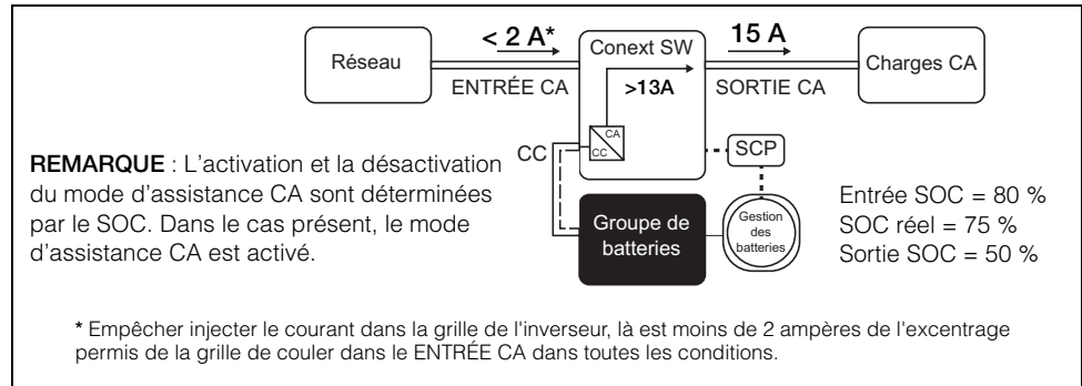
Figure 1-3 Mode d'assistance CA sur la base du SOC
