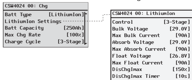
Figure 4-7 Écran du menu LithiumIon Settings (Paramètres LithiumIon)
