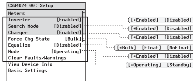
Figure 3-8 Menu Setup (Paramétrage) du Conext SW -Paramètres de fonctionnement
