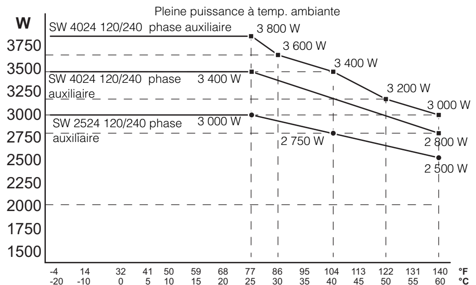
Figure 6-1 Courbe puissance de sortie vs réduction de température
