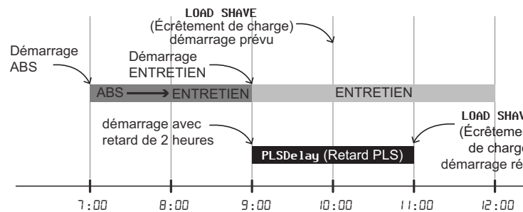
Figure 1-7 Exemple d'écèlement de charge avec retard de 2 heures
