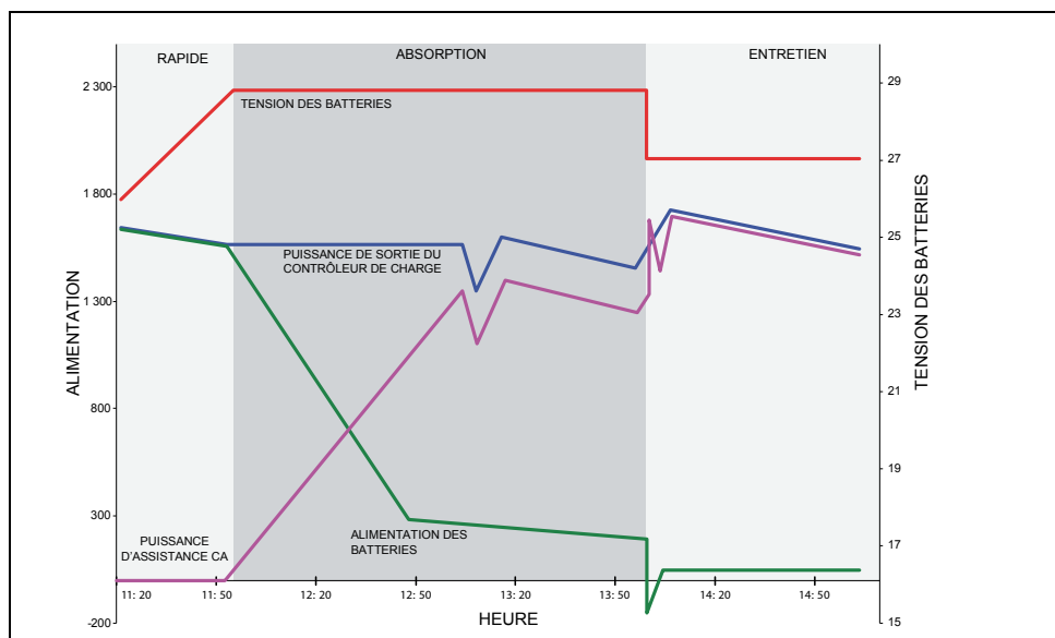
Figure 1-5 Cycle de charge avec assistance CA améliorée
