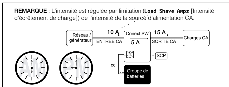
Figure 1-2 L'écrêtement de charge en action
