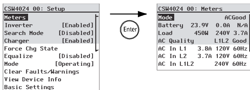
Figure 3-6 Lecture de l'écran Meters (Jaugeurs)
