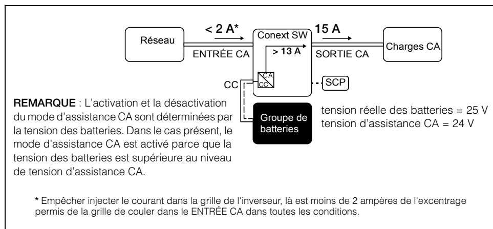
Figure 1-6 Assistance CA normale sans équipements Xanbus
