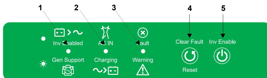
Figure 2-3 Boutons et voyants d'état du panneau frontal
