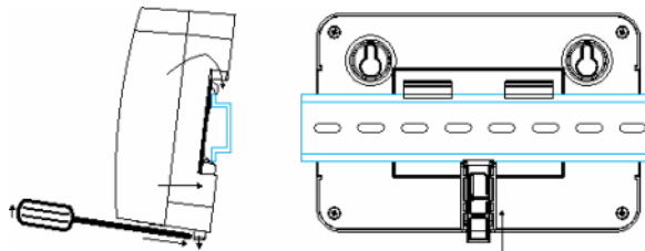
DIN rail catch
