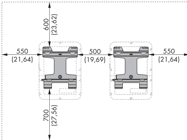
Figure 6 : Distances recommandées (Dimensions en mm (in))
