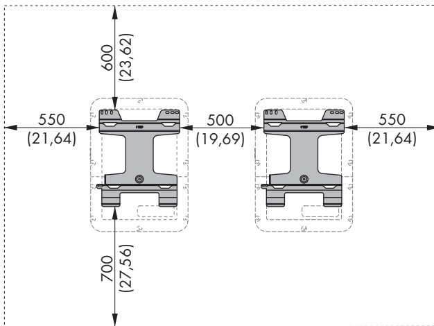
Imagen 6 : Distancias recomendadas (Medidas en mm (in))
