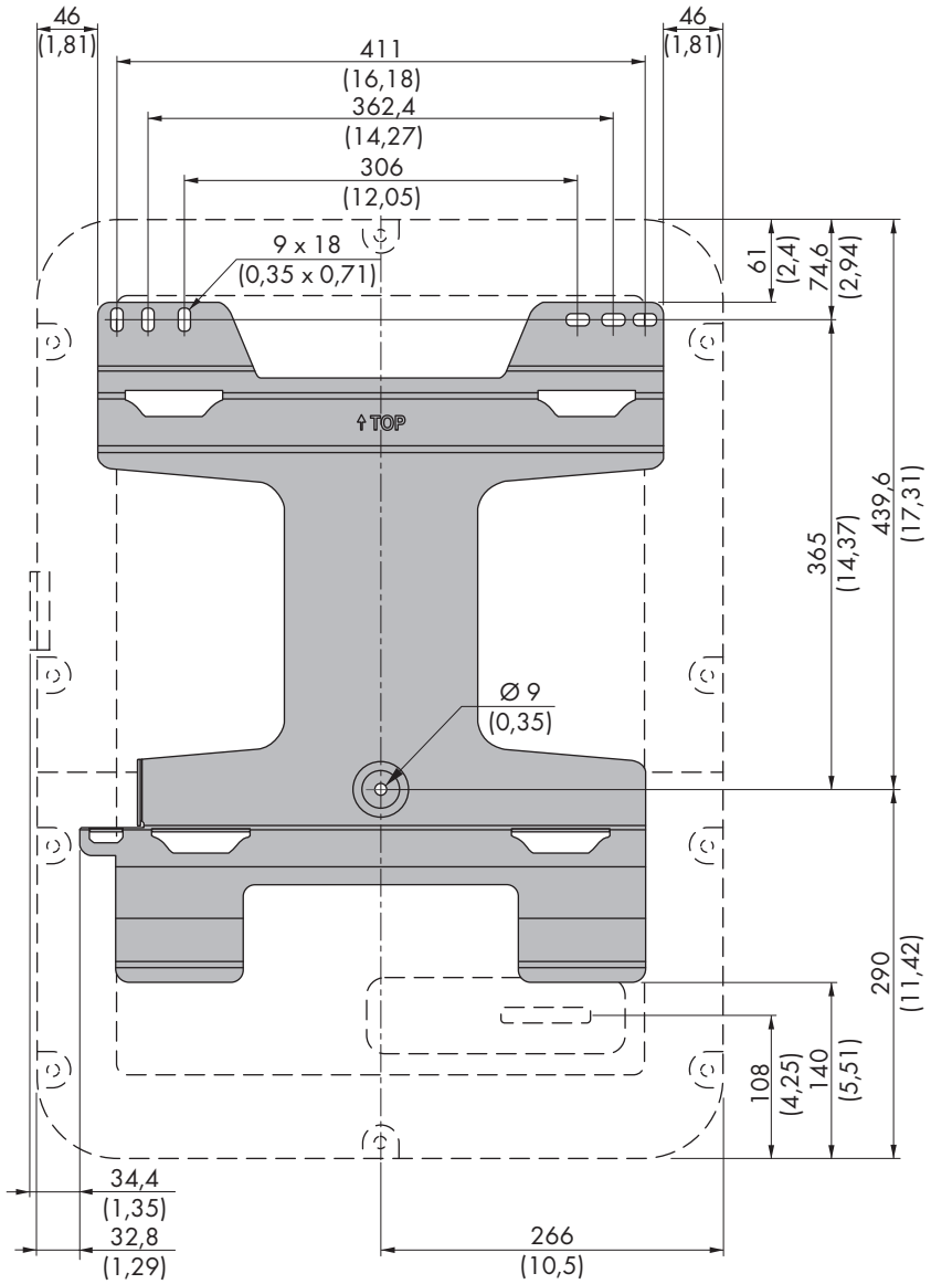
Figure 5 : Position des points de fixation (Dimensions en mm (in))
