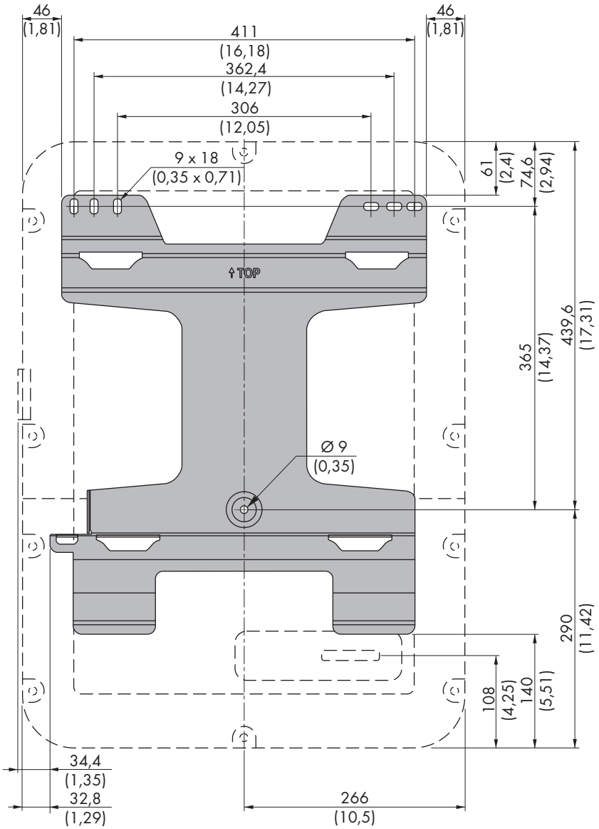
Imagen 5 : Posición de los puntos de fijación (Medidas en mm (in))
